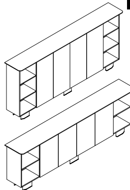
C5 | L*W*H 277 44 91 277 44 128
